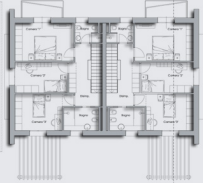
pianta piano primo
