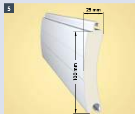
Profilo AW 100
