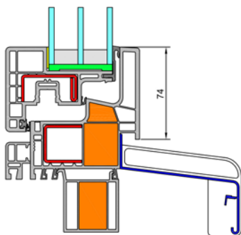
Schnitt Fußpunkt
