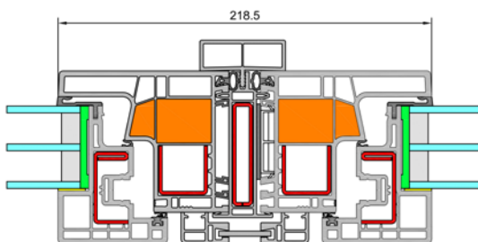
Schnitt Statikkopplung
