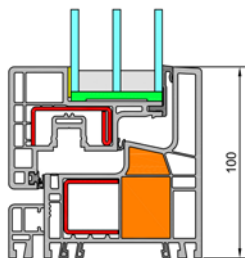
Grundschnitt GEALAN-KUBUS®
