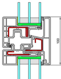
Schnitt Stulp/Pfosten
