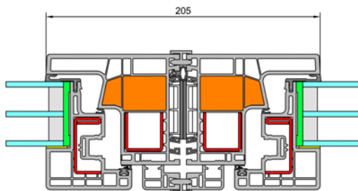
Schnitt Kopplung
