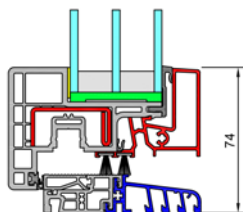
Schnitt Fenstertür
